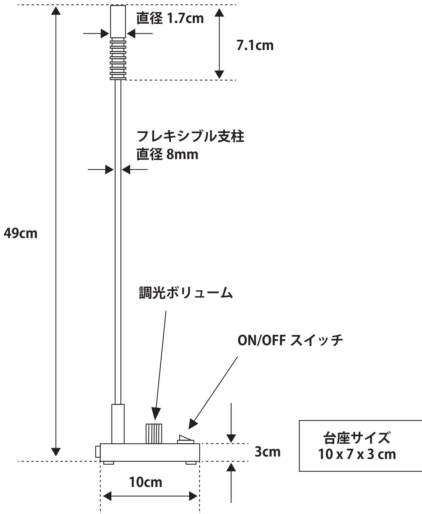
支柱を伸ばした状態の寸法 (フレキシブルアームは 2 灯)
